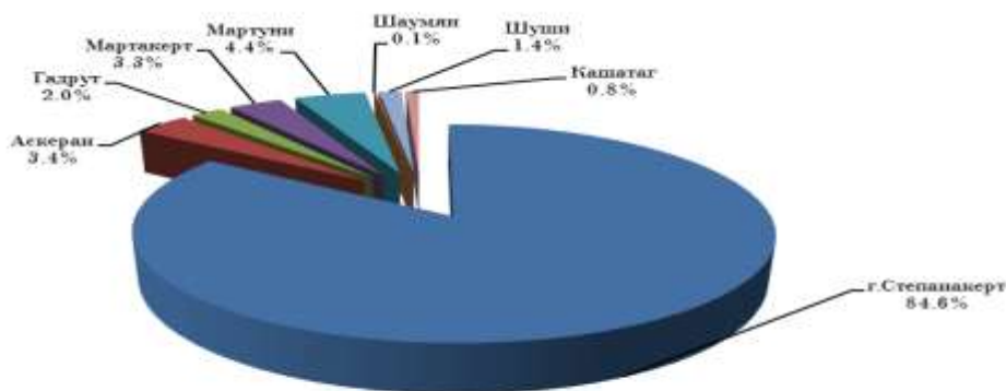
Распределение объема услуг по районам АР, в процентах за январь- декабрь 2018г.,%
