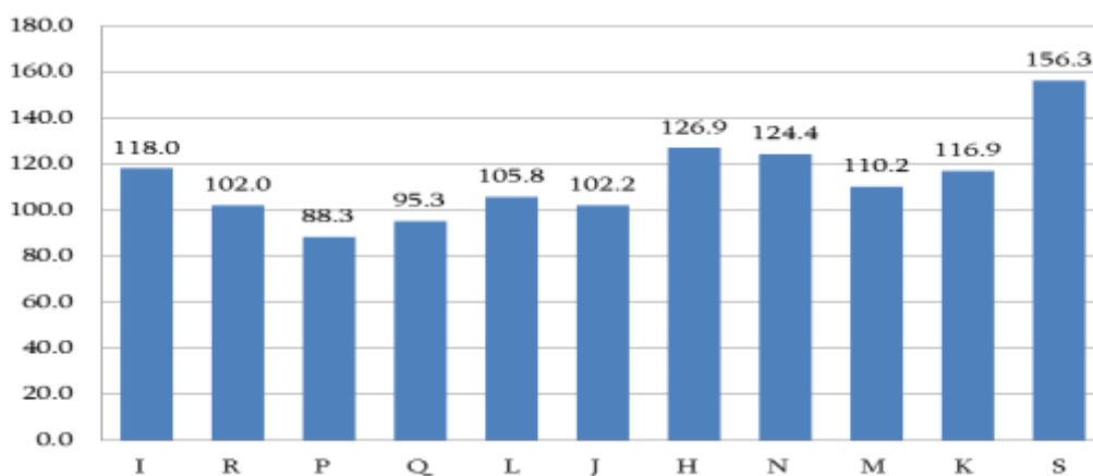
Индексы объема услуг, за январь- декабрь 2018г, к соответствующему периоду предыдущего года, %
