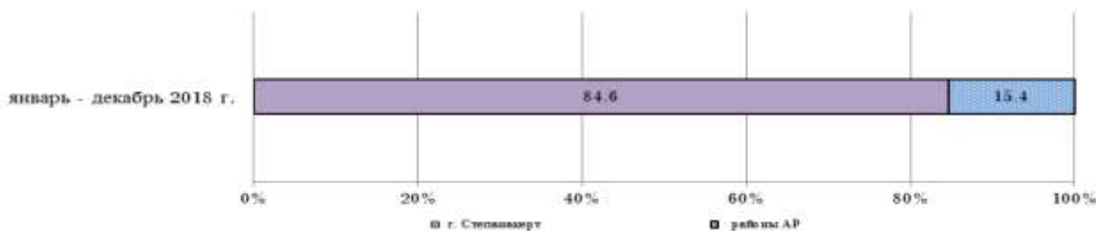
Объем услуг по г. Степанакерту и другим районам АР, %
