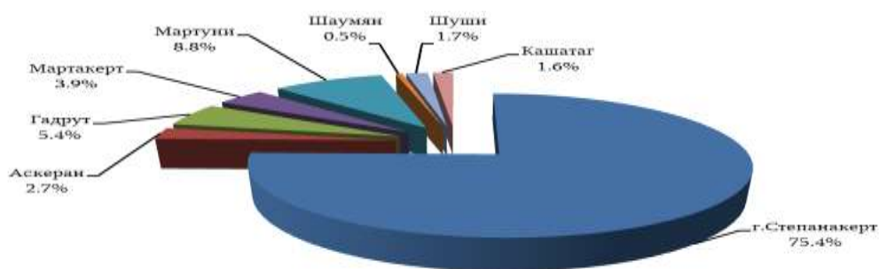
Структура оборота торговли по районам, за январь- декабрь 2018г., %
