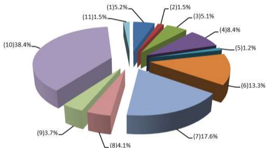
Структура услуг, за январь- декабрь 2018г. (%)
